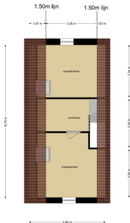
Plattegrond tweede verdieping
