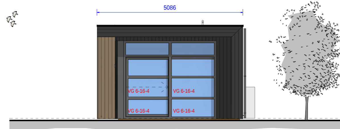
RECHTERZIJGEVEL
