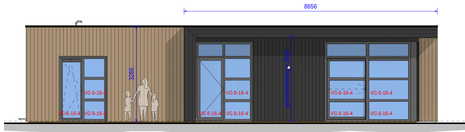
VOORGEVEL
