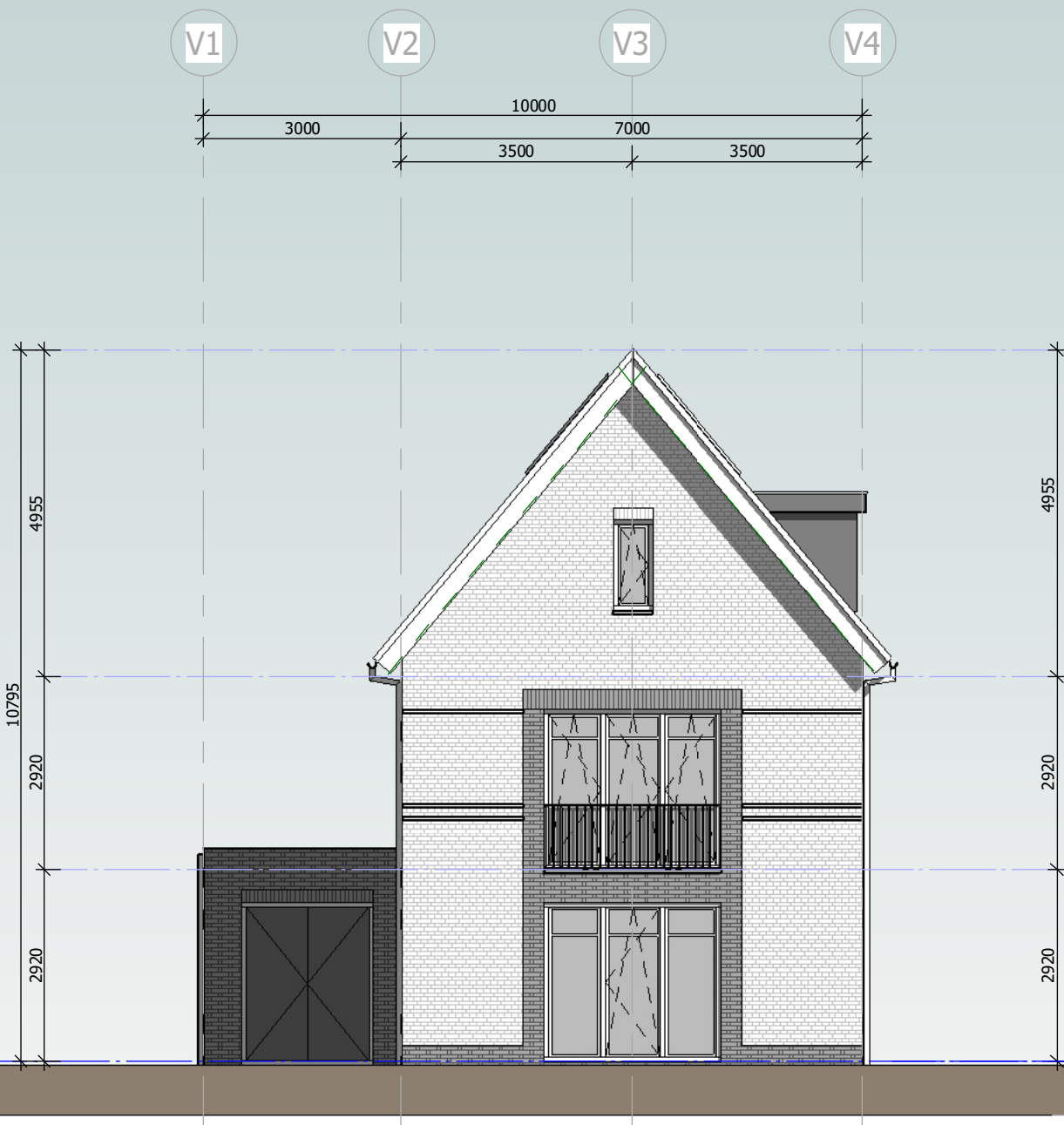
voorgevel vrijstaand (1:100)
