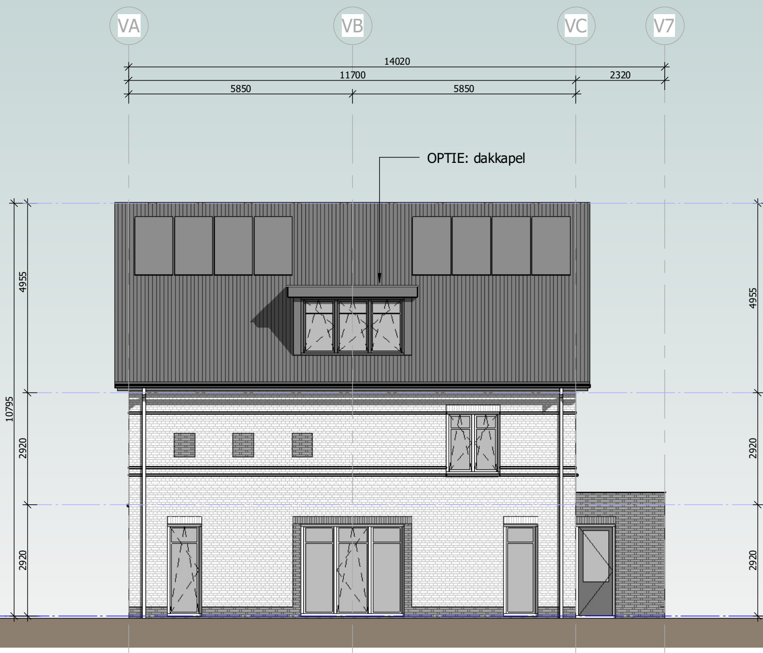
rechter zijgevel vrijstaand (1:100)
