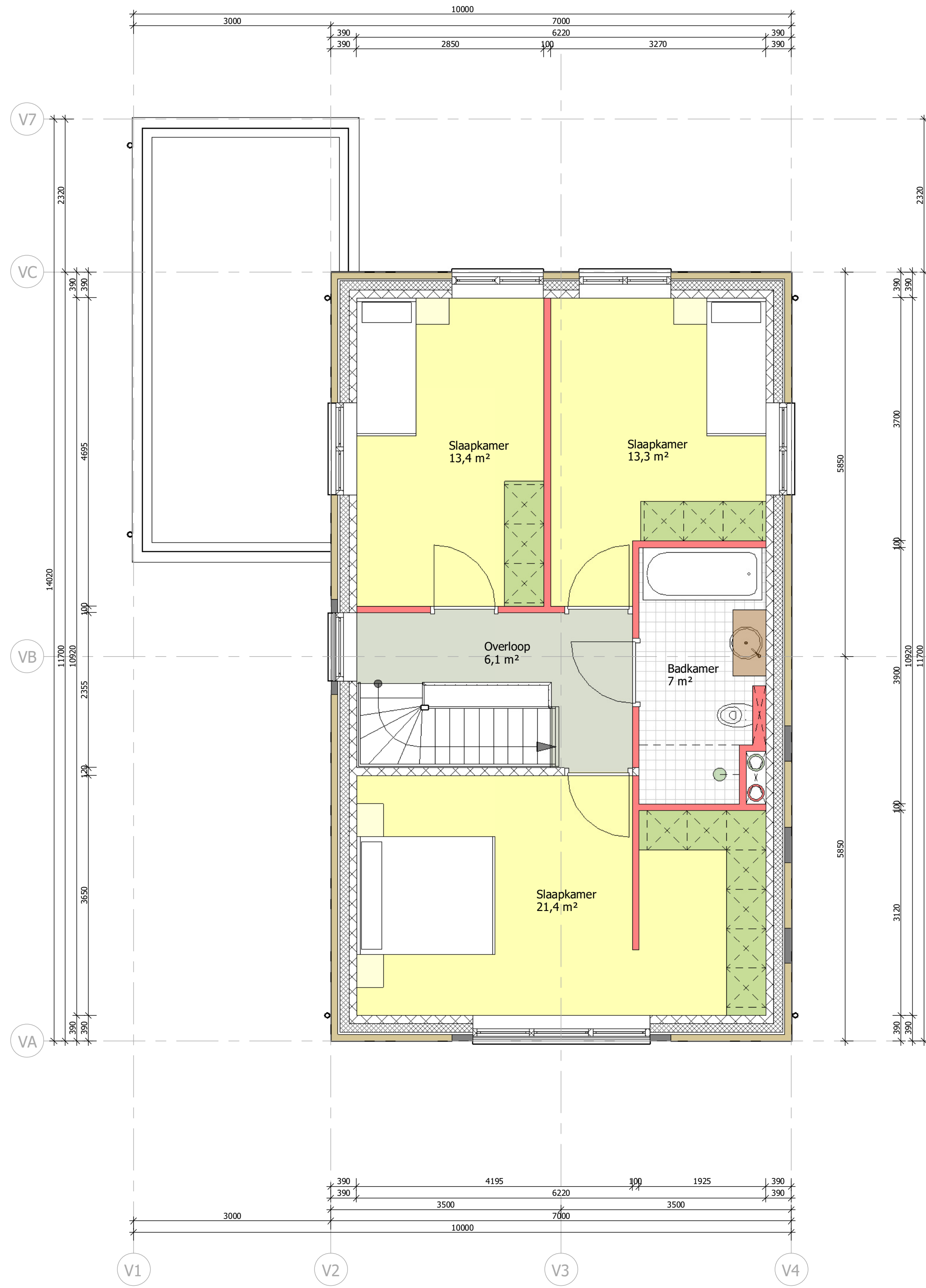
1e verdieping (1:50)
