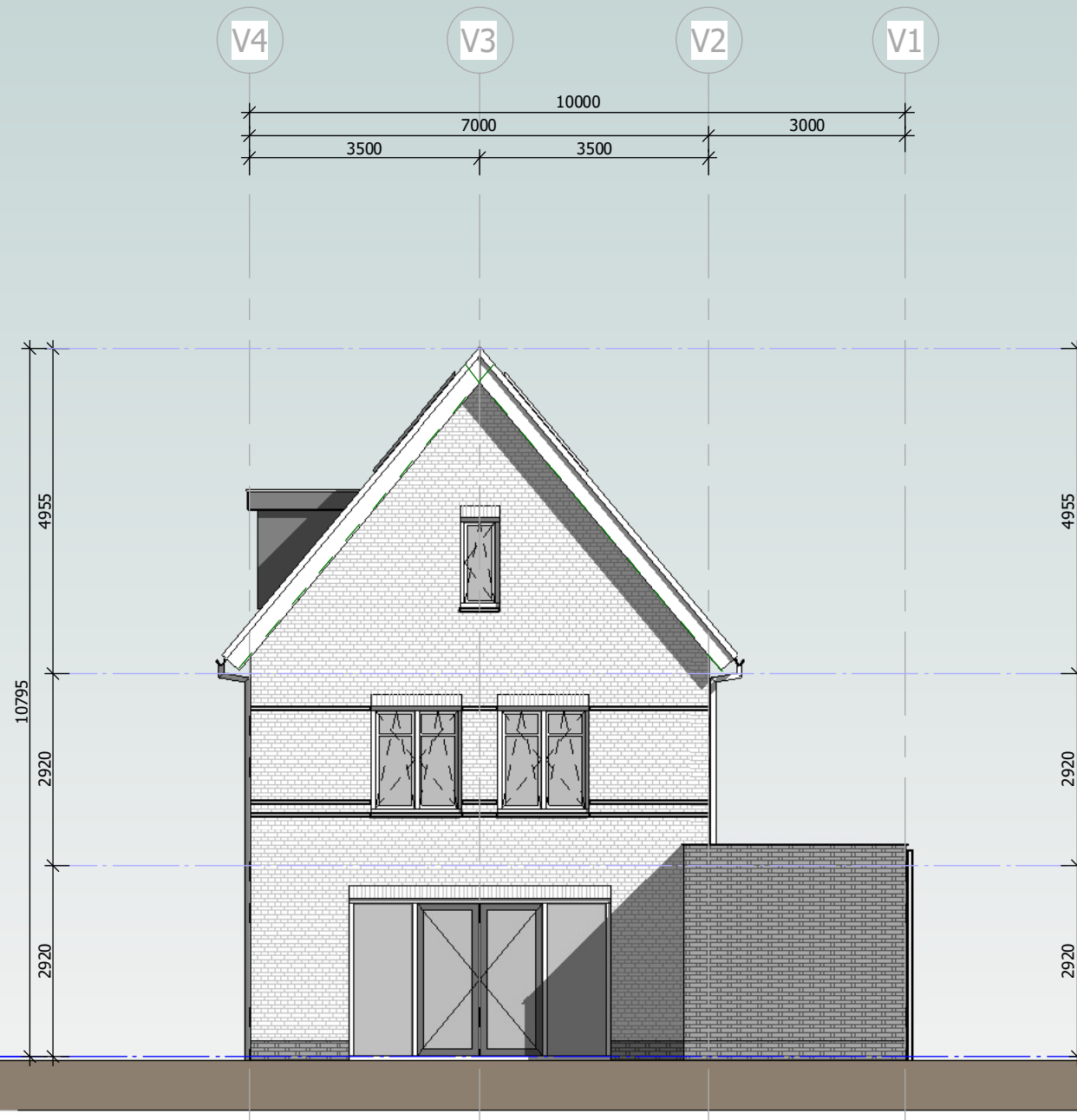
achtergevel vrijstaand (1:100)
