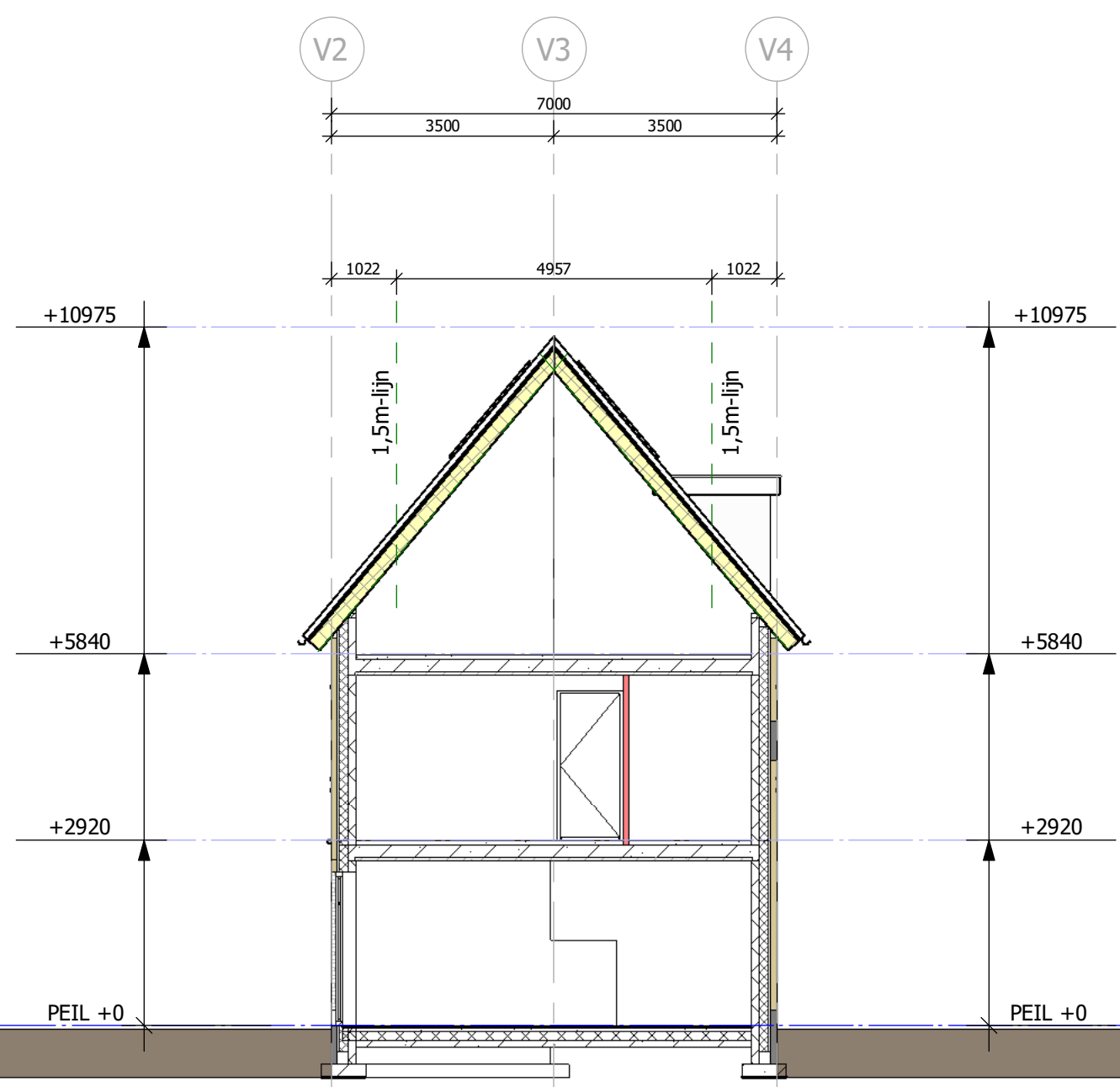
doorsnede V-V (1:100)
