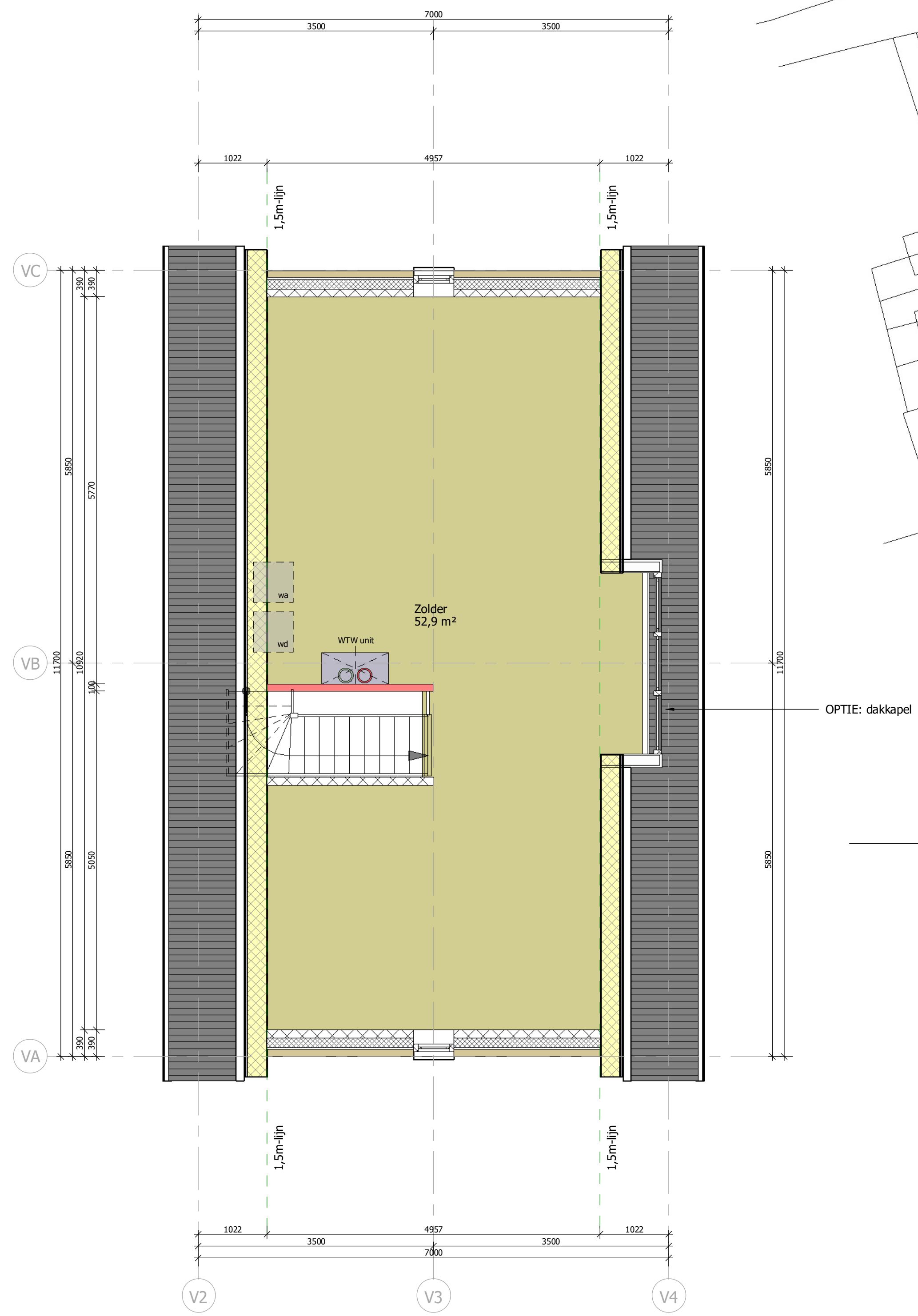
2e verdieping - (1:50)
