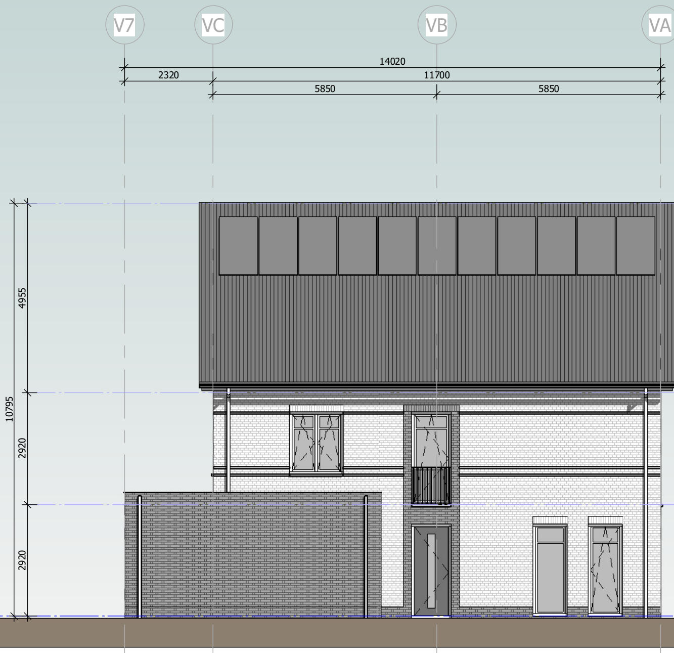
linker zijgevel vrijstaand (1:100)
